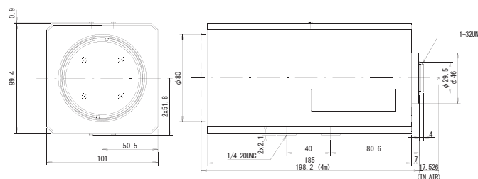
寸法
