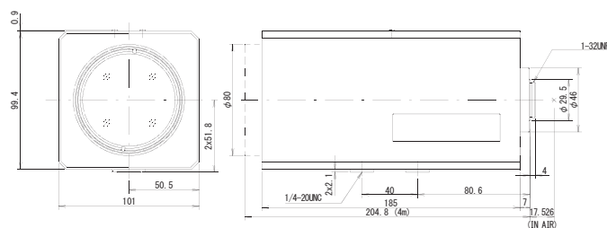
寸法
