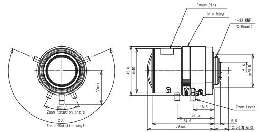
寸法
