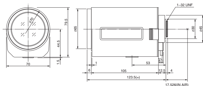
单位:mm
