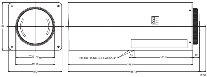
寸法
