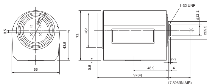
寸法
