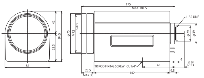
寸法
