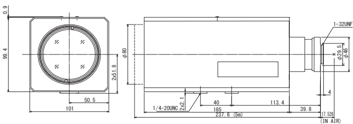
寸法
