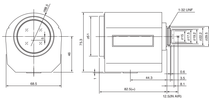
寸法
