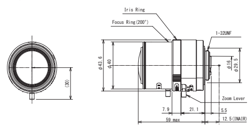
寸法
