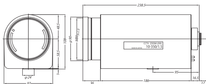
寸法
